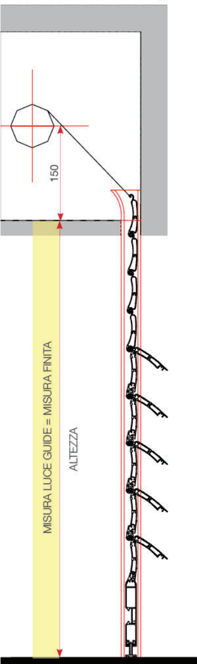
Sez. Verticale Fig. 5
